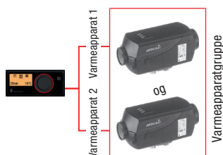
Bilde 6: EasyStart Pro med 2 luftvarmere i én gruppe
