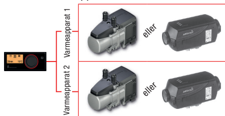
Bilde 4: EasyStart Pro med 2 separate styrbare varmeapparater
